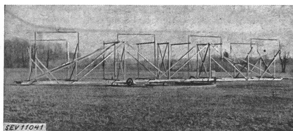
Fig. 6. Drehbare Richtantenne der Bell-Telephon-Laboratorien in Holmdel, New York
