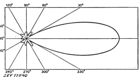
Fig. 5. Strahlungsdiagramm der Richtantenne
