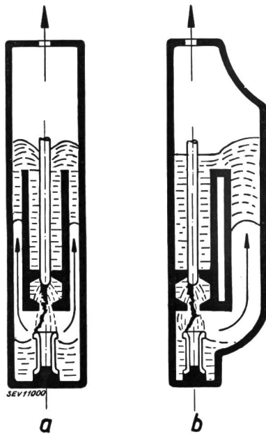
Fig. 1. Vergleich der neuen Führung von Gas und Öl (b) mit der bis- herigen (a)
