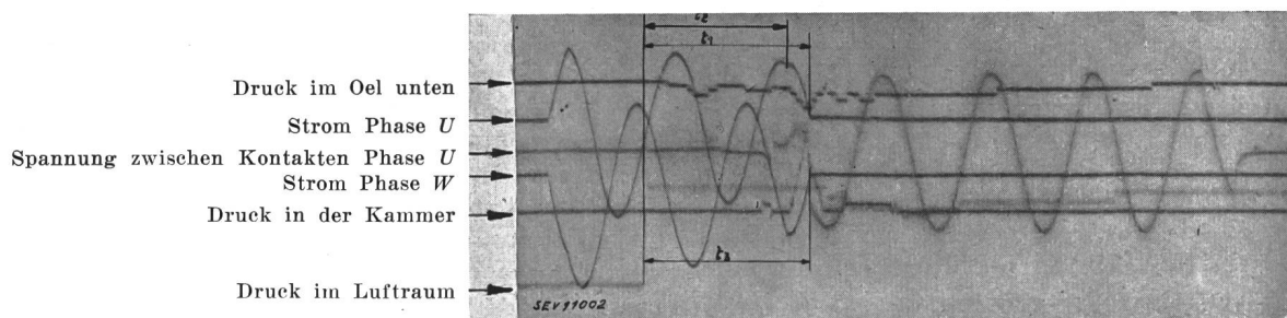
Fig. 3. Oszillogramm einer Abschaltung von 5800 A unter 23 kV mit einem Ölstrahlschalter 20 kV, 600 A
