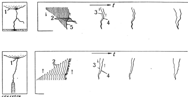
Fig. 8. Blitzbildung über der Ebene und am hohen Turm (Wolkenkratzer). Links: Bild mit ruhender Kamera. Rechts: Bild mit Boys-Kamera (Mc Eachron). t Zeit. 1 Negative Ladung. 2 Leuchtende Enden des ersten Leitblitzes. 3 Leitblitz eines Teilblitzes. 4 Hauptblitz eines spätern Teilblitzes. 5 Hauptblitz des ersten Teilblitzes (fehlt bei der Blitzbildung aus der Turmspitze).
