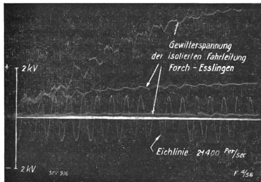
Fig. 11. Beispiele atmosphärischer Ueberspannungen auf 1200-V-Fahrleitung Spannungsanstieg während ca. 10^{-3} Sekunden (Gewittermessungen 1928).
