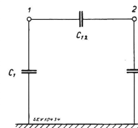
Fig. 1. Ersatzschema benachbarter Uebertragungsleitungen.
