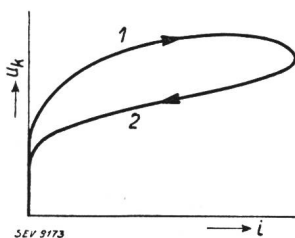
Fig. 4. Spannung-Strom-Charakteristik. 1 Stossanstieg. 2 Stossrückgang.
