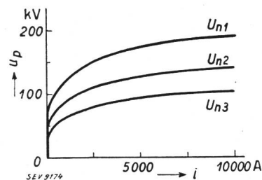
Fig. 5. Restspannung-Strom-Charakteristik. U_{n1}...U_{n3} Nennspannung des Ableiters. i Stoßstrom. u_p Restspannung.
