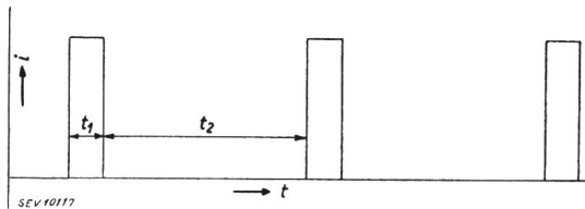
Fig. 1. Prinzipielle Form des Impulses.
