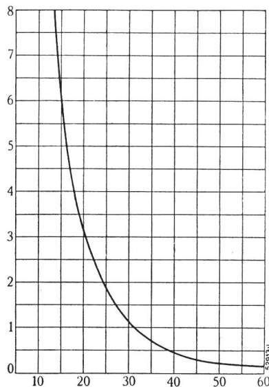
Fig. 1. Beziehung zwischen Anlagekosten und Störungsanfälligkeit von Leitungen Abszisse: Anlagekosten in 1000 Fr. pro km. Ordinate: Störungsanfälligkeit = Anzahl Störungen pro Jahr auf 100 km Leitungslänge. Die Verminderung von Störungen auf Leitungen, d. h. die Erhöhung ihrer Betriebssicherheit, erfordert vergrößerte Anlagekosten.
