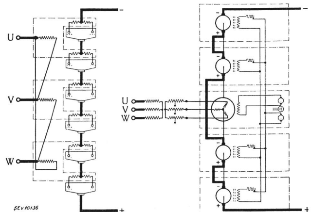
Fig. 15. Vergleich einer grossen Mutatoreinheit mit einer Maschineneinheit
