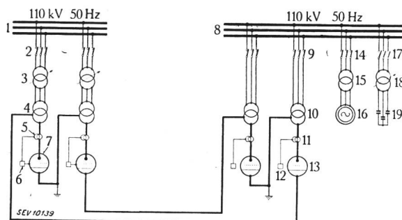
Fig. 18. Prinzipschema einer Gleichstrom-Übertragungsanlage Links: Sendestation. Rechts: Empfängerstation.
