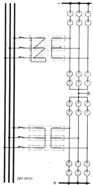
Fig. 13. Grosse Doppel-Einheit in Grätz-Schaltung für 500 A, 2 \times 200 kV, 200 MW.
