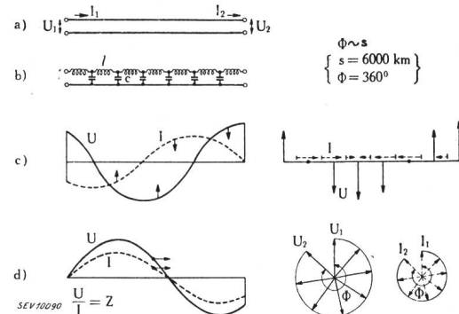
Fig. 2. Die physikalischen Vorgänge auf einer verlustlosen langen Leitung.
