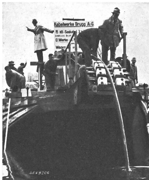
Fig. 9. Verankerung des Kabels in Wädenswil.
