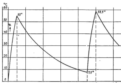
Erwärmung bei kurzzeitigem Betrieb (30 min mit 4 h Pause), KA, 5,1 kW dauernd, 1400 U/min, tropfwassergeschützt, belastet mit 7,3 kW.
