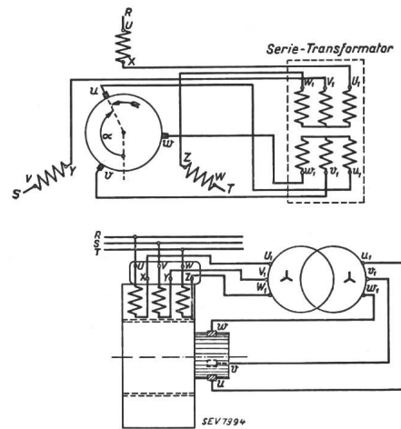
Fig. 7. Drehstrom-Serie-Kommutatormotor (Prinzipschema).
