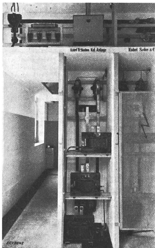
Fig. 4. Emissions-Transformatoren 2000 V.
