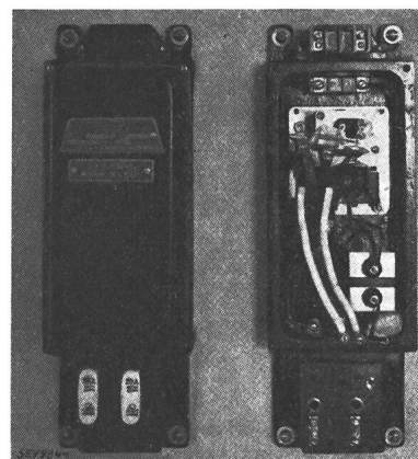
Fig. 5. Emissions-Transformatoren 16 000 V.
