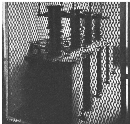
Fig. 5. Emissions-Transformatoren 16 000 V.
