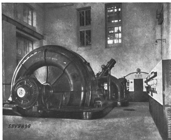
Fig. 6. Lötschwerk. 12 000-kVA-Drehstromgenerator 8.
