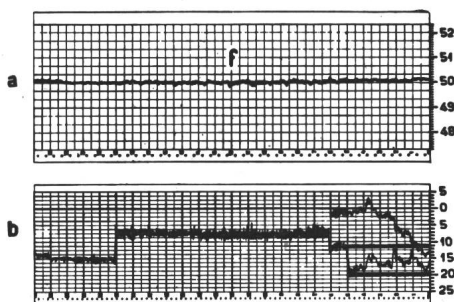
Fig. 4. Uebergabeleistung (Handregulierung). + bedeutet Lieferung - bedeutet Bezug
