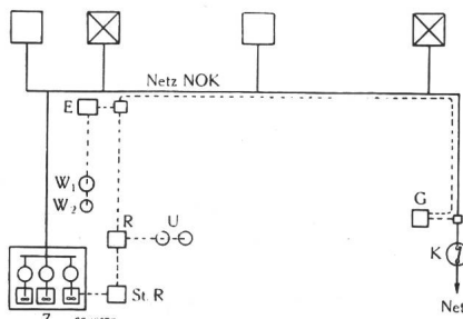
Fig. 11. Schematische Darstellung der Fernregulierungsanlage im Überlandnetz.
