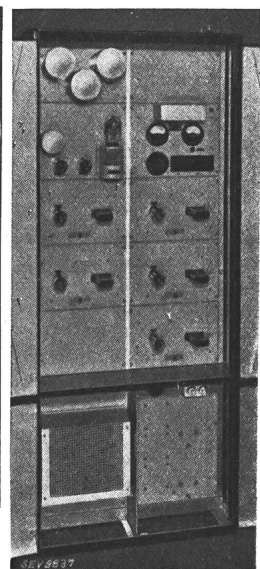
Fig. 7. HF-Fernmessempfänger.
