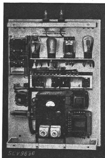
Fig. 6. HF-Sender für Trägereastung.
