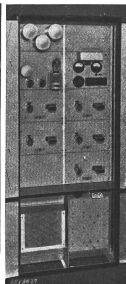
Fig. 7. HF-Fernmessempfänger.
