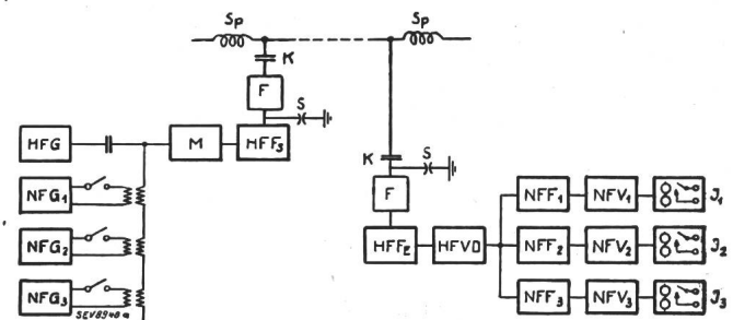
Fig. 4. Uebersichts-Schaltbild einer Mehrfach-Fernmessanlage. HFG HF-Generator NFG 1...3 NF-Generatoren M Modulations- und Endstufe HFF s HF-Sendefilter F Koppelfilter Sp HF-Sperre HFF e HF-Empfangsfilter HFVD HF-Verstärker und Demodulator NFF 1...3 NF-Filter NFV 1...3 NF-Verstärker mit Pegelregler und Gleichrichter J 1...3 Impuls-Empfänger S Spannungableiter K Kopplungskondensator
