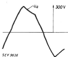
Osz. 7. Erzeugte Wechselspannung, U_{\sim}/U_{\sim} = 0,96 , Z\omega C = 0,89 , \cos \varphi = 1 .
