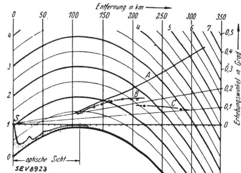
Fig. 4. Profilschnittdarstellung zum Vergleich des gerechneten und gemessenen Strahlen- verlaufs. Sender B, \lambda = 7,17 m. S Sender, A gerechneter Verlauf, B, C ge- messener Verlauf des untersten Maximums des Vertikaldiagramms. Die Rechnung gilt für geradlinigen Strahlenverlauf. Messungen am 30. 9., 3. 8., 11. 10. 1935.
