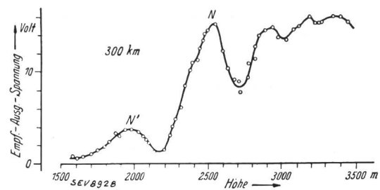
Fig. 9. Gemessene Vertikaldiagramme. (Sender N, \lambda = 4,1 m) 12. 7. 1935.
