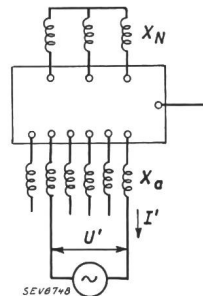
Fig. 3. Schaltbild für den einachsigen Kurzschlussversuch.
