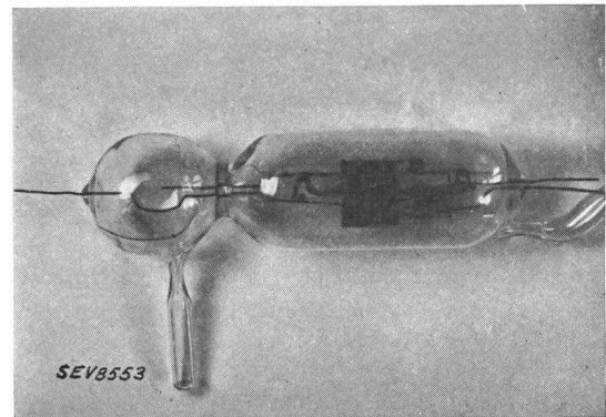
Fig. 4. Elektrostatisches Relais mit aufgebauter Ionisationskammer.
