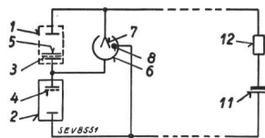
Fig. 2. Prinzipisches für Feuermelder.
