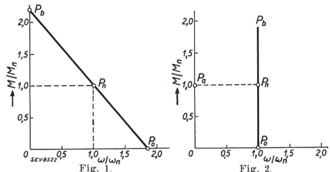
Fig. 1. Schematisierte Reihenschluss-Charakteristik. Fig. 2. Schematisierte Nebenschluss-Charakteristik.
