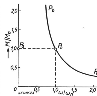
Fig. 3. Idealer Gleichstrom-Reihenschlussmotor.
