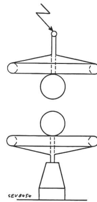
Fig. 4. Geschirme Kugelfunkenstrecke.
