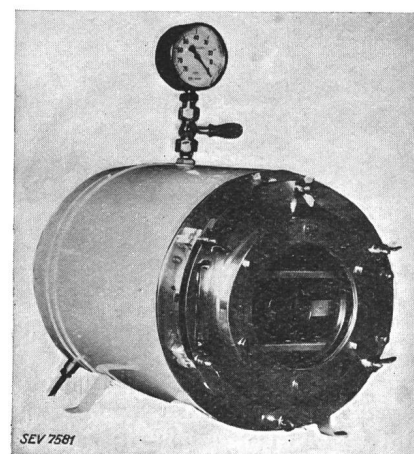
Fig. 8. Laboratoriums-Vakuumschrank.
