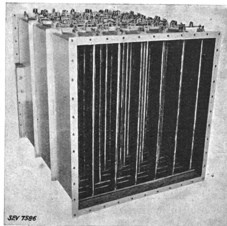
Fig. 13. Lufterhitzer, 100 kW.
