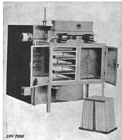
Fig. 12. Konditionierschrank (Rückseite).
