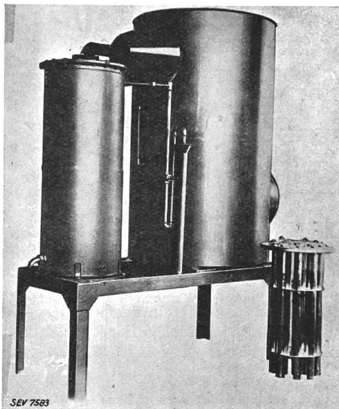
Fig. 10. Destillierapparat 50 kW.
