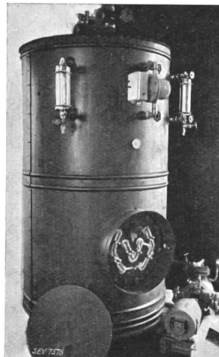
Fig. 2. Akkumulierdampfkessel.
