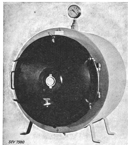
Fig. 7. Laboratoriums-Vakuumschrank.
