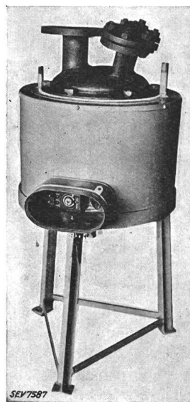
Fig. 14. Klein-Autoklave
