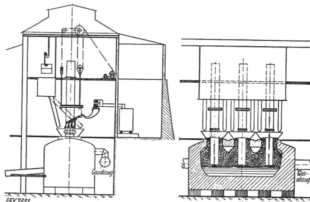
Fig. 2. Tysland-Hole-Ofen.
