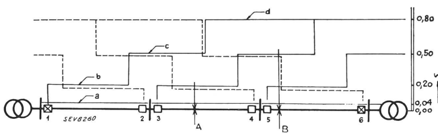
Fig. 1. Anwendung der unverzügten automatischen Wiedereinschaltung auf eine mittels Distanz-Relais geschützte, in mehrere Abschnitte unterteilte Uebertragungsleitung. a Kennlinie der Schnellauslösung der Schalter 1 und 6. b, c, d Auslösekennlinie der Distanzrelais. 1 und 6 Schalter mit Schnellauslösung und automatischer Wiedereinschaltung. 2 bis 5 Schalter ohne Schnellauslösung und ohne automatische Wiedereinschaltung.
