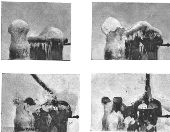
Fig. 31. Oeffnung eines vereisten Trennkontaktes. Ausschnitte aus einer Filmaufnahme.
