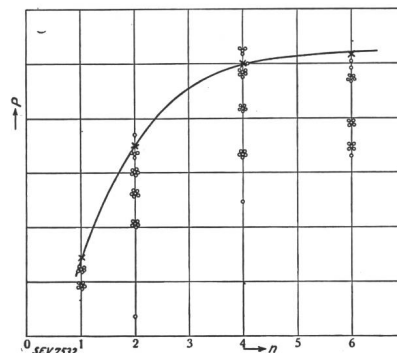
Fig. 25. Abschaltleistung in Abhängigkeit der Unterbrechungsstellenzahl bei Höchstspannungen. ○ gute Abschaltungen. × Schaltungen mit Stehlichtbogen. Die entsprechenden Versuche wurden bei gleichbleibendem Totalluftverbrauch durchgeführt.
