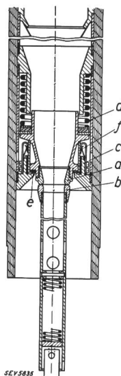
Fig. 15 Düsenkontakt.
