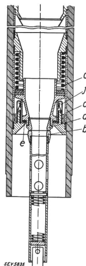
Fig. 15 Düsenschnellkontakt.
