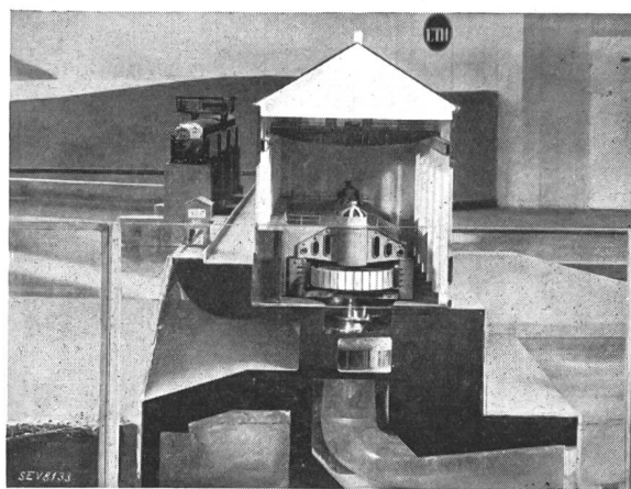
Fig. 7. Maschinenhaus des Niederdruckwerkes.
