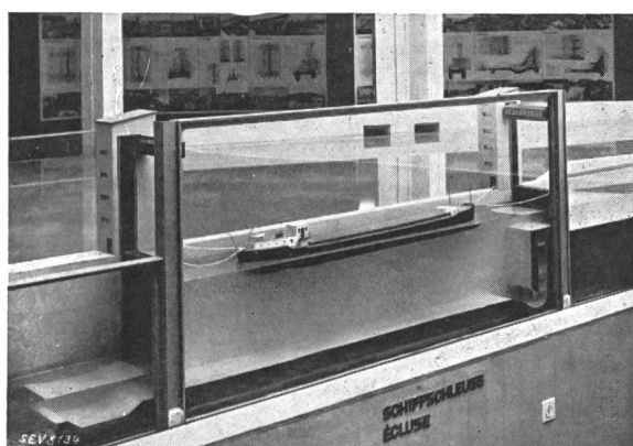
Fig. 8. Schiffschleuse beim Niederdruckwerk.
