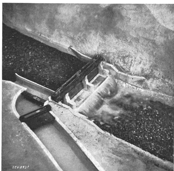
Fig. 5. Wasserfassung zum Mitteldruckwerk.
