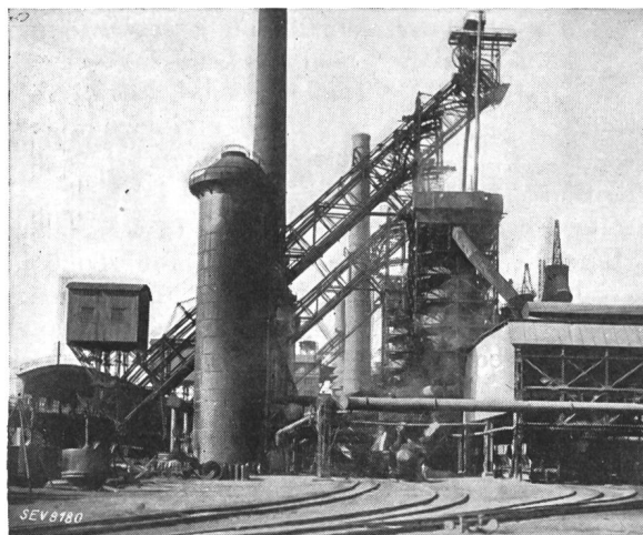
Fig. 1. Hochofenanlage.
