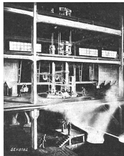
Fig. 4 (rechts). Elektrische Niederschachtofenanlage.
