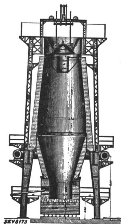
Fig. 1. Kokshochofen, schematischer Schnitt.
