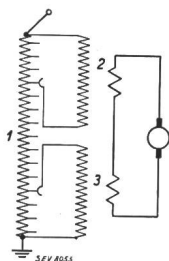
Fig. 3. Schaltprinzip der Hochspannungssteuerung. 1 ein Transformator mit Anzapfungen. 2, 3 zwei gleiche Transformatoren ohne Anzapfungen auf gemeinsamem Eisenkern.
