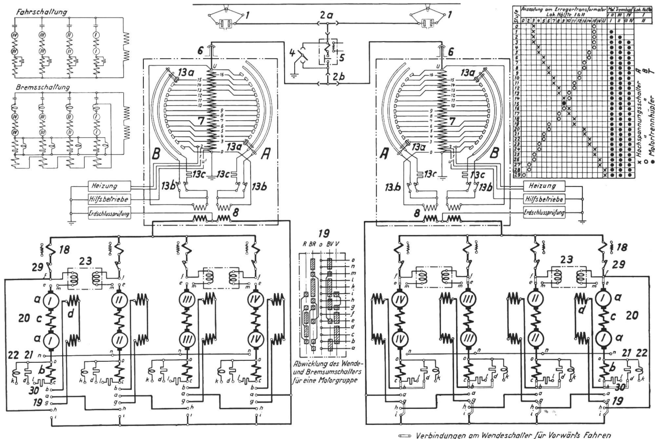
Fig. 2. Hauptstromkreise.
