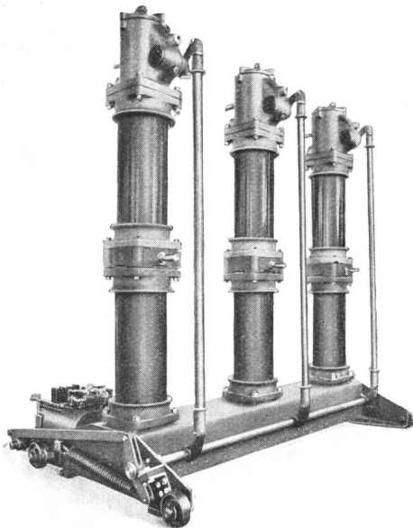
Oelstrahlsschalter der Sprecher & Schuh A. G.
