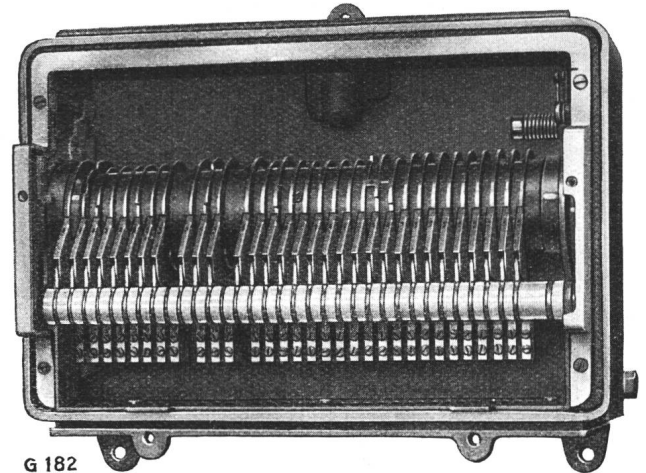
G 182 Steuerschalter der Ghilmetti & Cie. A. G. für komplizierte Schaltprogramme.
