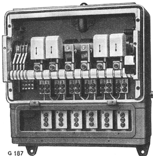
G 187 Dreipoliger Fernschalter 120 A der Ghilmetti & Cie A. G.
