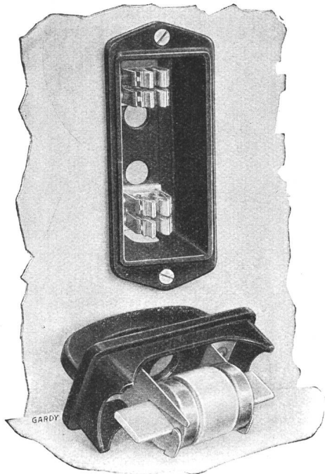
Gardy-Versenk-Hochleistungssicherung.
