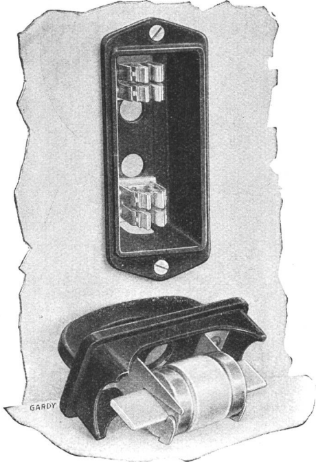
Gardy-Versenk-Hochleistungssicherung.
