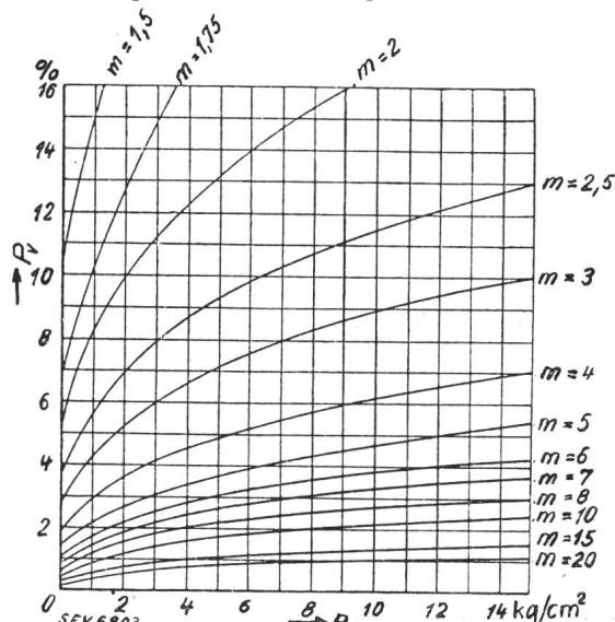
Fig. 2. Verlust P_v (in %) in Funktion des Kesseldruckes p (in \text{kg}/\text{cm}^2 ), für verschiedene Werte von m .
