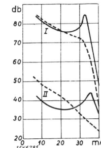
Fig. 3. Verzerrungs-Verminderung durch Gegenkopplung im Verstärker Fig. 2 gegenüber der Grundharmonischen, in Funktion des Ausgangsstromes. I { ——— 2. Harm. } mit Gegenkopplung. { - - - - 3. Harm. } II { ——— 2. Harm. } ohne Gegenkopplung. { - - - - 3. Harm. }
