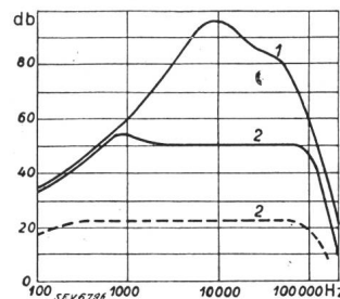
Fig. 4. Frequenzgang des Verstärkers Fig. 2 ohne und mit zwei verschieden starken Gegenkopplungen, 1 ohne, 2 mit Gegenkopplung.
