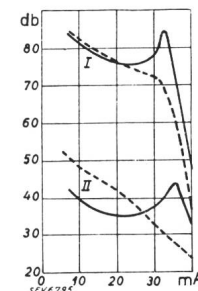
Fig. 3. Verzerrungs-Verminderung durch Gegenkopplung im Verstärker Fig. 2 gegenüber der Grundharmonischen, in Funktion des Ausgangsstromes. I { — 2. Harm. } mit Gegenkopplung. { - - - 3. Harm. } II { — 2. Harm. } ohne Gegenkopplung. { - - - 3. Harm. }
