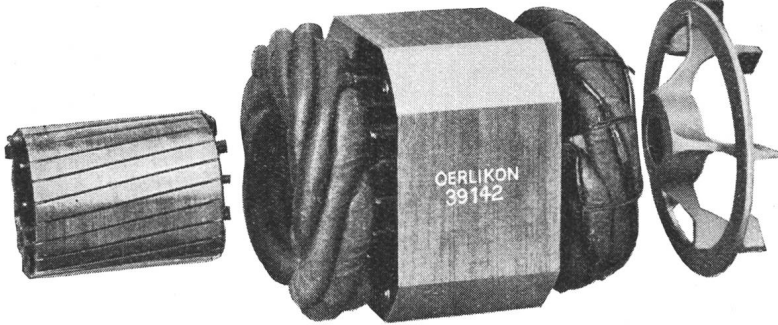
MFO-Einbaumotor, bestehend aus genietetem und bewickeltem Stator, Rotor und Ventilator.
