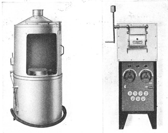
Four à bain de sel de la S. A. Four Electrique, Delémont.
