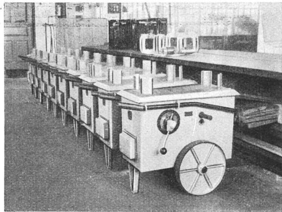
Schweissgruppen der Firma Truninger.
