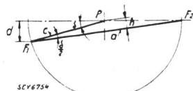
Fig. 6. Einhebelssystem (mit Zugfeder).
