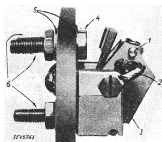
Fig. 10. Schaltelement des Zentrifugalanlagers Roulland 1935. 1 Knopf zum Regulieren der Federspannung. 2 Verbindungskabel. 3 Zentrifugalkontaktstück. 4 Kontaktstück. 5 Isolation aus Mica. 6 Anschlüsse der Widerstände.
