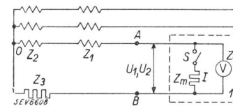
Fig. 3. Ersatzbild der Messung. Z_1 + Z_2 + Z_3 = Z_n = Netzimpedanz. 1 Messinstrument.
