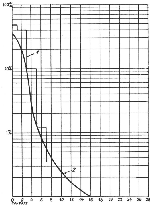
Fig. 4. Relative Anzahl der Beobachtungen in % in Funktion der Kursabweichung in Graden. 1 kurze Wellen. 2 lange Wellen.
