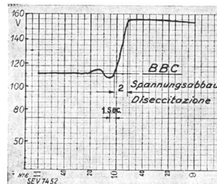
Fig. 5. Hochleistungs-Schnellregler.
