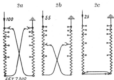
Fig. 2. Schematische Wicklungsanordnung einer regulierbaren Oerlikon-Erdschlüsspule.
