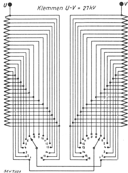
Fig. 3. Verbindungsschema einer in 16 Stufen regulierbaren Oerlikon-Erdschlüsspule, mit Parallelschaltung pro Säule.
