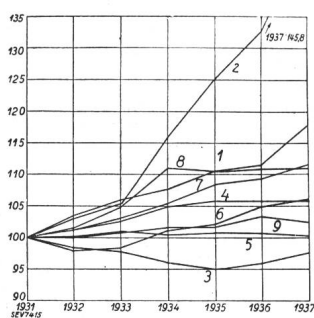
Fig. 3. Evolution de la puissance unitaire par appareil de 1931 à 1937. (1931 = 100.)
