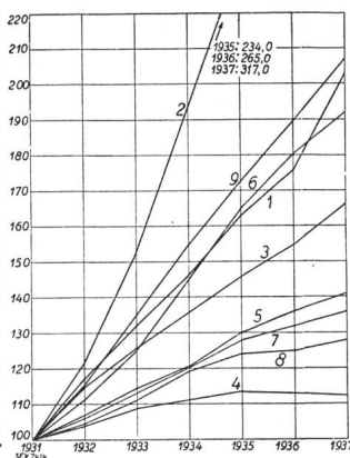
Fig. 2. Evolution de la puissance installée de 1931 à 1937. (1931 = 100.)
