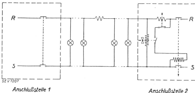
Fig. 7. Fernsteuerungsschaltung bei parallelgeschalteten Glühlampen.
