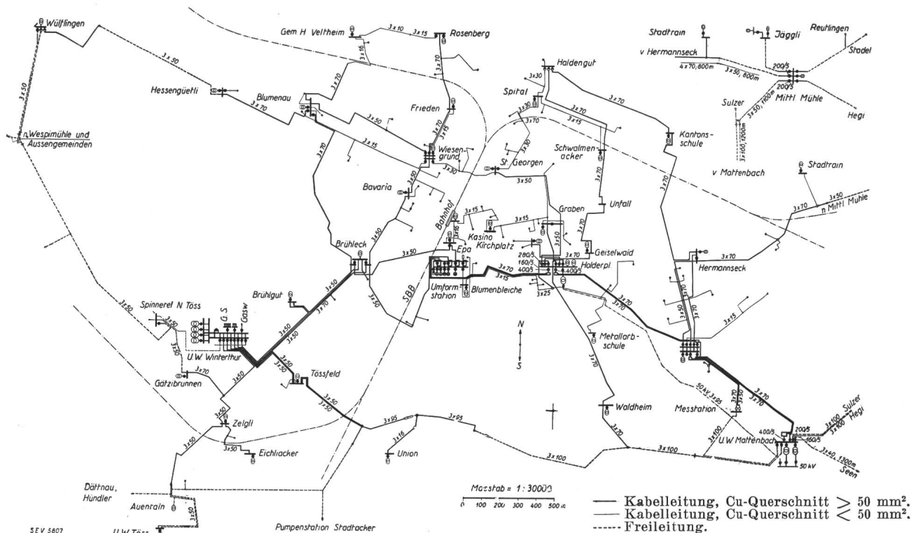
Fig. 5. 3 kV-Netz des EW Winterthur (gegenwärtiger Stand). Die grossen Punkte bedeuten Schalter mit Relaisschutz und die kleinen Punkte Abonnentenstationen.
