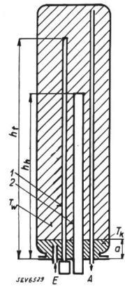
Fig. 1. Speicher mit erster Kaltwas- serschicht. E Einlauf, A Aus- lauf, 1 Thermo- stat, 2 Heize- element.
