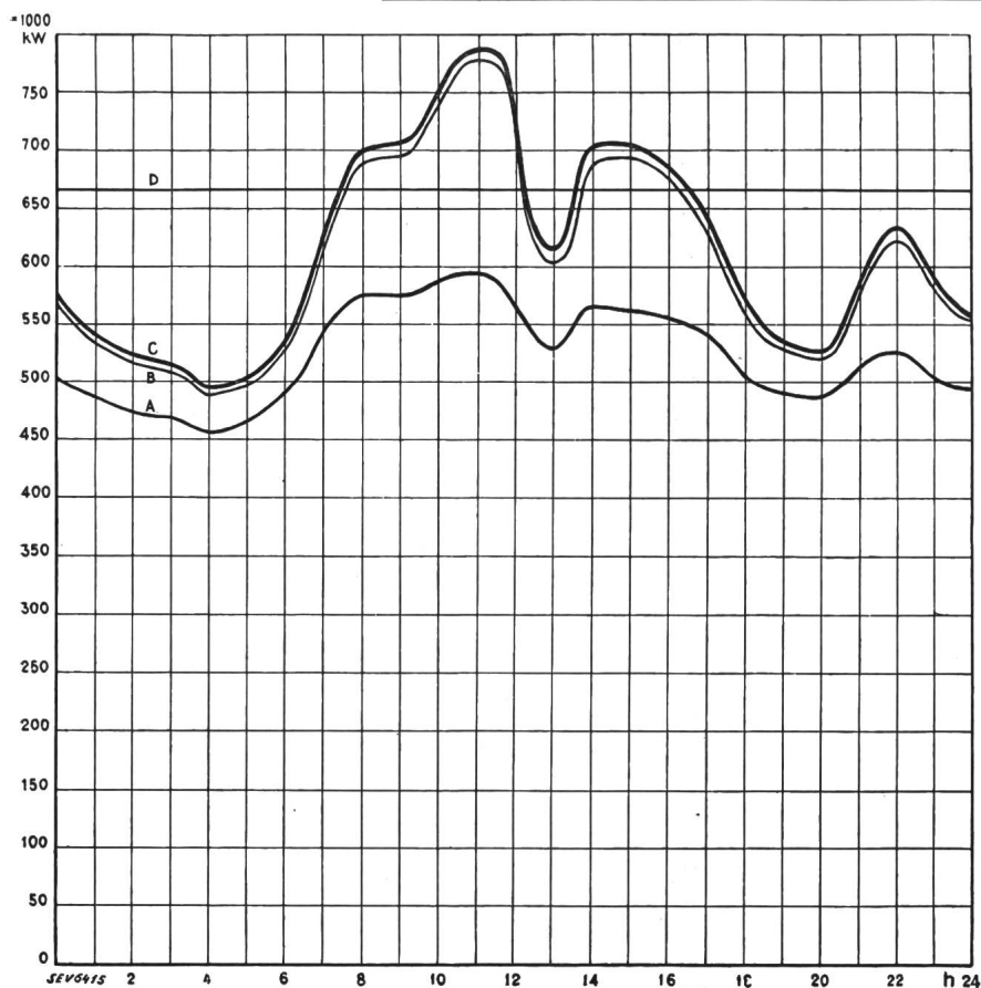
Diagramme de charge journalier du mercredi 14 juillet 1937.
