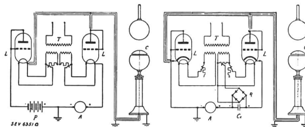
Fig. 1. Schéma pour la mesure de la haute tension par courant capacitif redressé. Montage Haefely.
