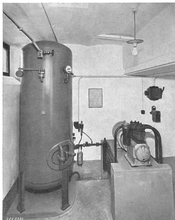
Fig. 9. Kompressor-Anlage.
