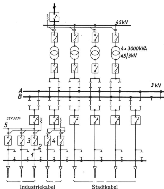
Fig. 1. Unterwerk Winterthur. Prinzip-Schema.
