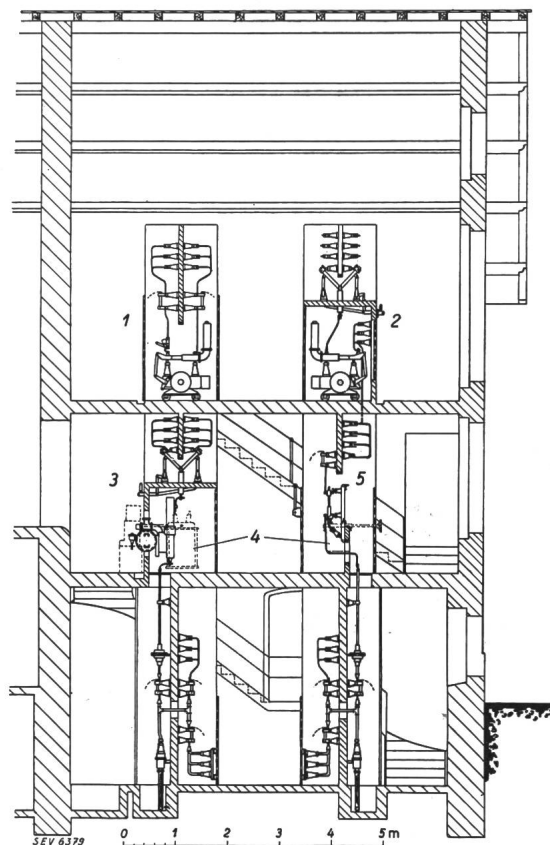
Fig. 2. Querschnitt des Schalthauses.
