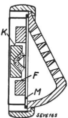
Fig. 1. Mikrofonkapsel Lorenz.
