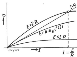
Fig. 1. Leerlaufkurven mit Widerstandsgerade.
