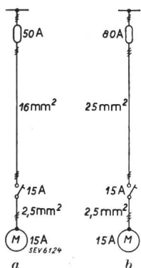
Fig. 8. Selektivität zwischen Querschnittsicherung und Selbstschalter. a Bei Verwendung von Selbstschalter mit thermischer Überstrom- und elektromagnetischer Schnellauslösung muss die Querschnitt-Sicherung für 50 A bemessen sein. b Bei Verwendung von Selbstschalter mit rein thermischer Überstromauslösung muss die Querschnitt-Sicherung für 80 A bemessen sein.
