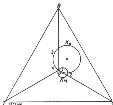
Fig. 2. Kreisdiagramm der Nullpunktverlagerung durch Netzunsymmetrie ( U_0 ) bei variabler Spuleneinstellung. Kreis K_0 vor der «Verdrillung», Kreis K_M nach der «Verdrillung» (Phasentausch in Streckenmitte).
