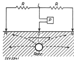
Fig. 1. «Dispositif différentiel.»
