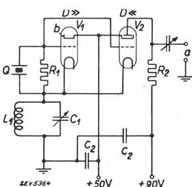
Fig. 8. Funktionsschema zu Fig. 7. V_1 Triodenteil der Tetrode, Durchgriff gross, Schirmgitter wirkt als Anode. V_2 Tetrode, Durchgriff klein.
