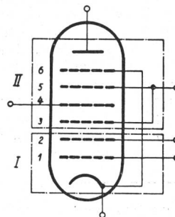
Fig. 2. Oktode
