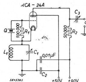
Fig. 7. Quarzgesteuerter Oszil- lator zur Erzeugung eines grossen harmonischen Spektrums. Q Quarz. R_1 = 100\,000\,\Omega ; R_2 = 50\,000\,\Omega ; C_1 = 100\,\text{pF} ; C_2 = 0,01\,\mu\text{F} ; C_3 = 50\,\text{pF} ; L_1 = \text{je nach Quarzfrequenz} .
