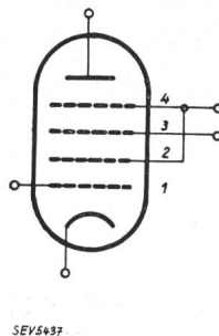
Fig. 1. Regelhexode
