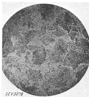
Fig. 4. Perlite dans de la ferrite.
