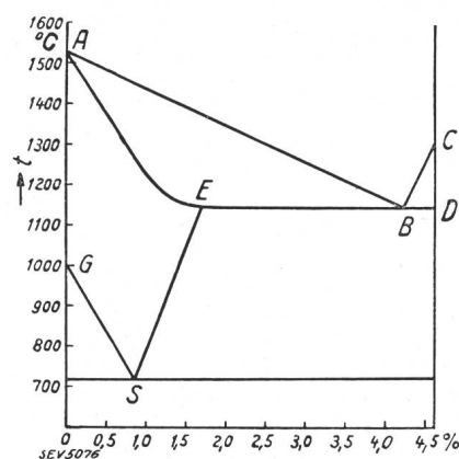
Fig. 1. Diagramme du système fer-carbone.
