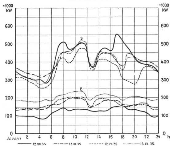
Fig. 7. Courbes de charge journalière de l'énergie livrée dans le pays et de l'énergie exportée.
